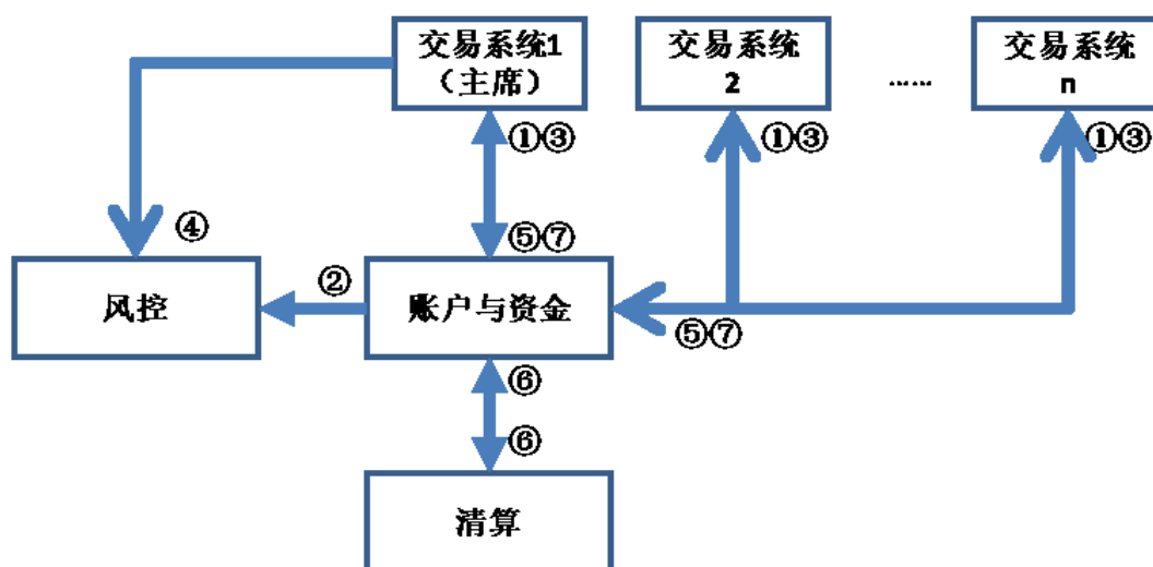
图1 期货公司柜台消息流示意图
